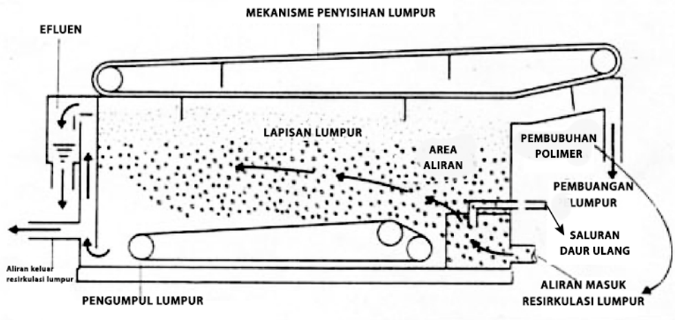
Gambar 56 Tipikal Unit Pengental Pengapungan ( Flotation Thickener )
