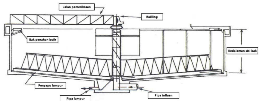
Gambar 29 Bak Pengendapan I dengan aliran radial
