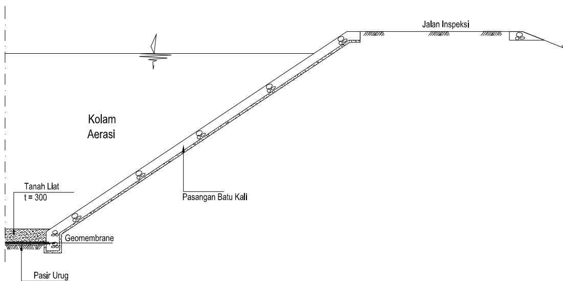
Gambar 59 Contoh Konstruksi Dinding Bangunan Kolam Pengolahan
